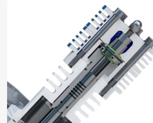
Quatrième étage en acier trempé avec 6 segments de piston en fonte spéciale
