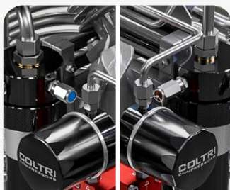
Válvulas de seguridad después de cada etapa de compresión
