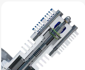
Cuarta etapa en acero templado con 6 anillos de pistón en hierro fundido especial
