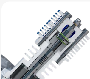
Cuarta etapa en acero templado con 6 anillos de pistón en hierro fundido especial
