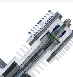
Cuarta etapa en acero templado con 6 anillos de pistón en hierro fundido especial
