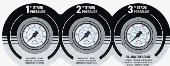
Manometri controllo interstadio
